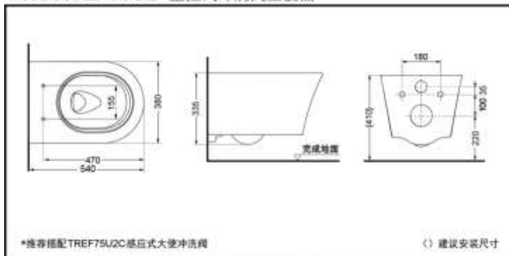
CW553RB-75U2 壁挂式冲洗阀坐便器
