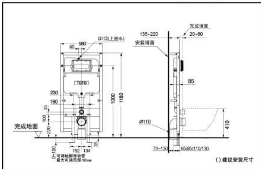
WH173B-562EB WH173B-572EB 手动隐藏式水箱
