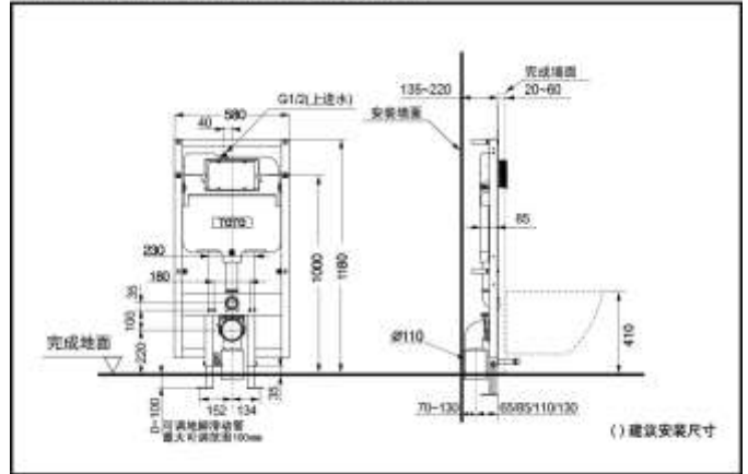
WH173BT-582EB 手动隐藏式水箱
