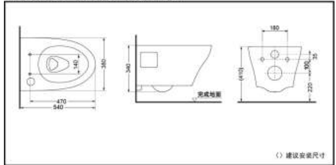
CW582EB 壁挂式隐藏水箱坐便器
