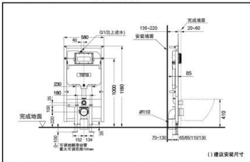
WH173B-822EB 手动隐藏式水箱
