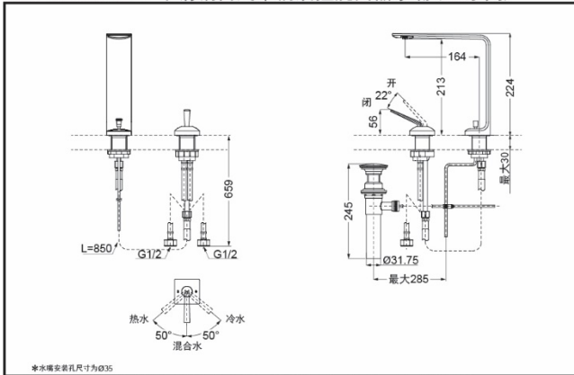
TLP02307B1 不锈钢台式单柄双控洗面器水嘴 (ZL系列)
