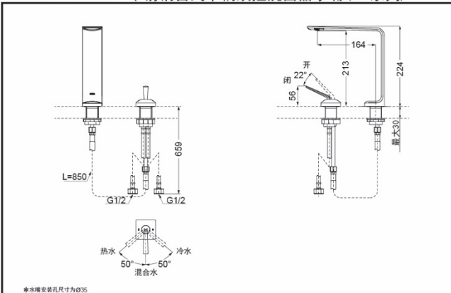
TLP02308B1 不锈钢台式单柄双控洗面器水嘴 (ZL系列)
