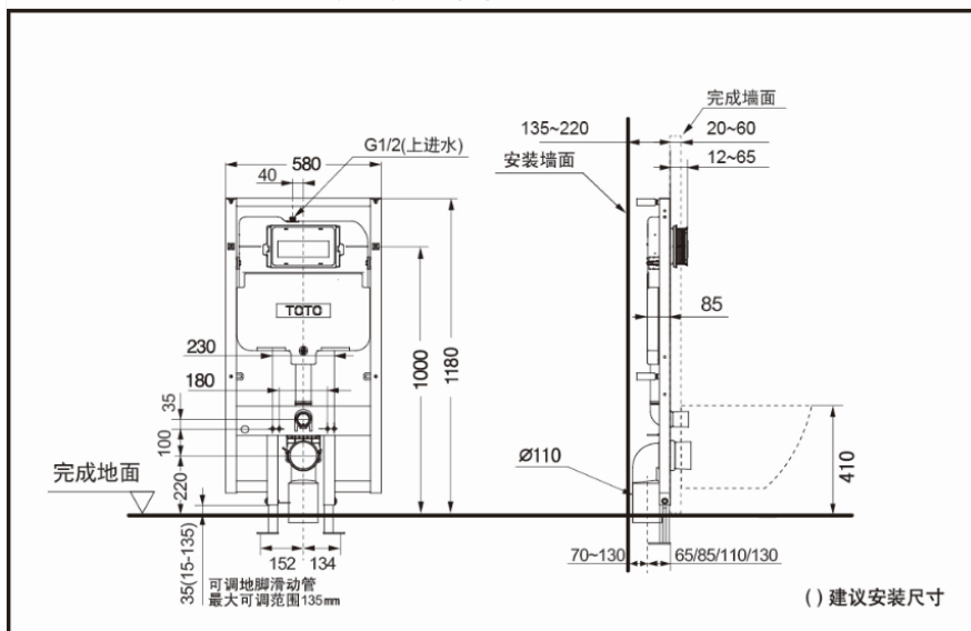
WH173B-822B 手动隐藏式水箱
