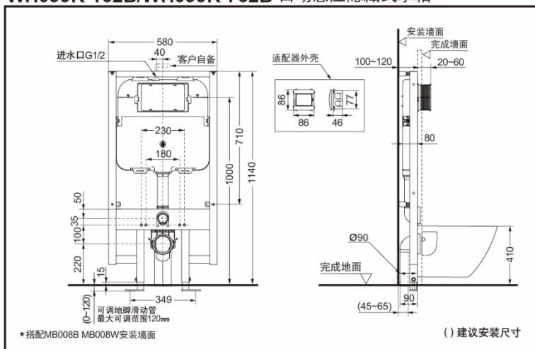
WH099R-162B/WH099R-762B 自动感应隐藏式水箱
